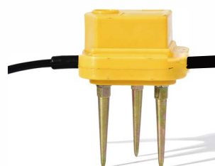
Geófono 3C terrestre
